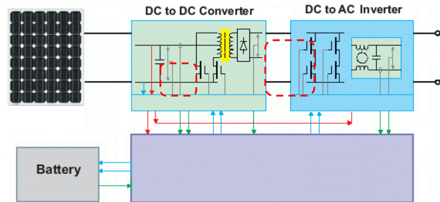
Converter/Inverter / BMS(電池管理系統)
